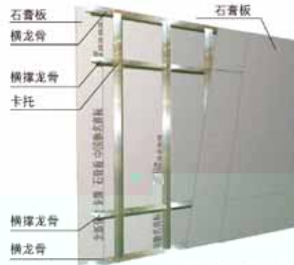
无贯通龙骨隔墙示意图
